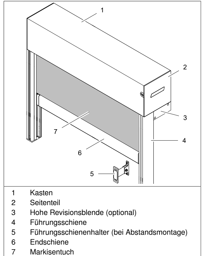
Abb. 1: Teileübersicht Vorbau-Markise mit easyZIP-Führung
